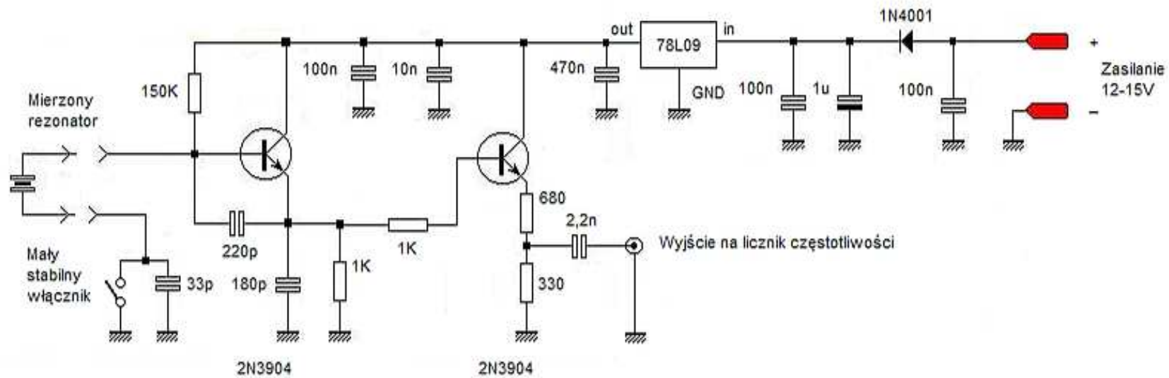
Układ do pomiarów i dobierania rezonatorów używanych do budowy filtrów kwarcowych
